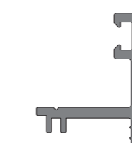
KAS 60 Stile Rebate
