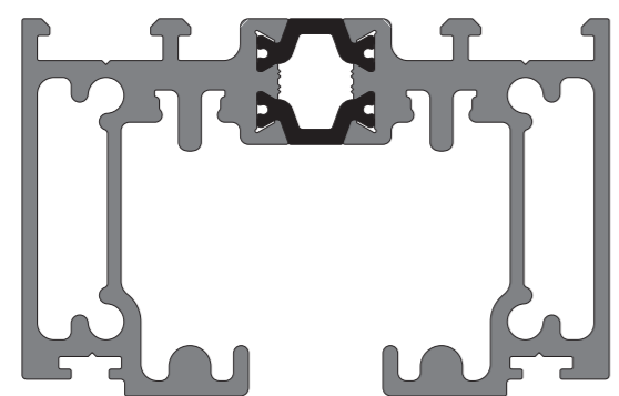
KAS 730 Header / Cill
