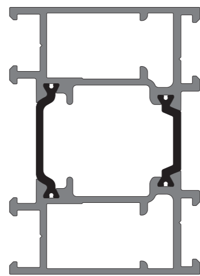
KAS 733 Jamb (4 Panel)
