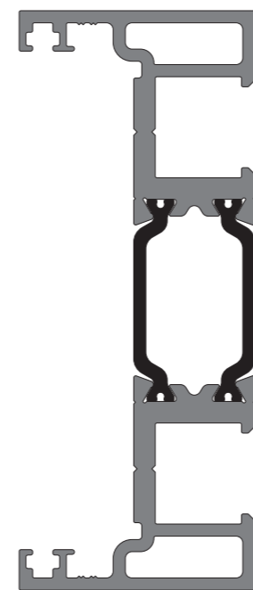
KAS 743 Adjustable Jamb Outer
